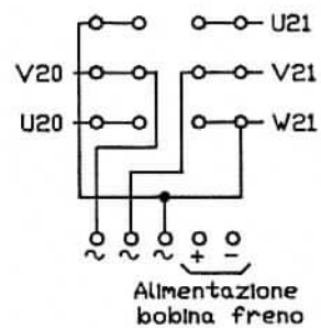
SCHEMA COLLEGAMENTO MORSETTIERA MOTORE (220V)
