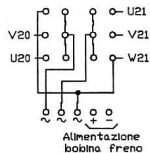
SCHEMA COLLEGAMENTO MORSETTIERA MOTORE (380V)
