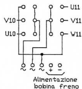
SCHEMA COLLEGAMENTO MORSETTIERA MOTORI (380V)
