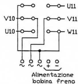
SCHEMA COLLEGAMENTO MORSETTIERA MOTORI (220V)
